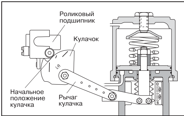
Рис . 4. Регулировка кулачка
